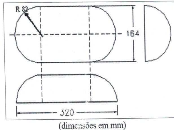
Figura 1: Aparatos de ensaio em formato de corpos cilíndricos para aplicação de força sobre a poltrona.
