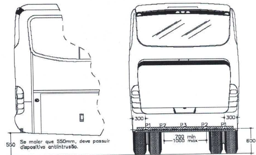
Figura 1: Dispositivo de proteção anti-intrusão traseiro.
