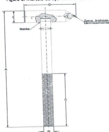
Figura 1: Martelo de aço ABNT 1010 ou 1020.
