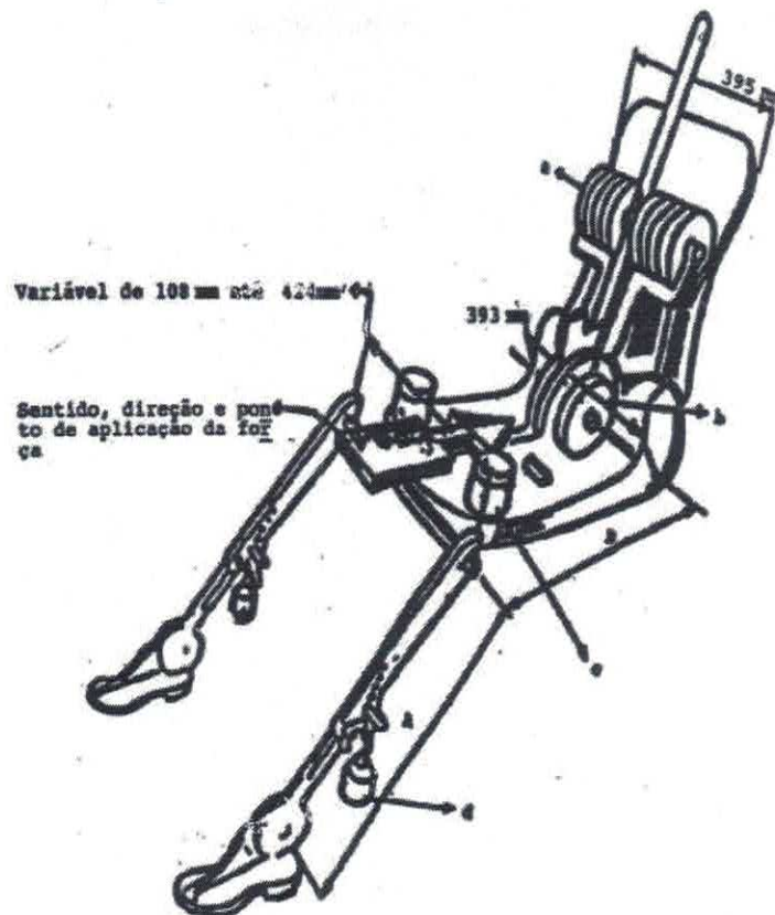
Figura 2: Dimensões do dispositivo tridimensional
