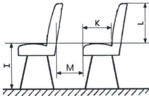
Figura 1: Dimensões referentes aos assentos
